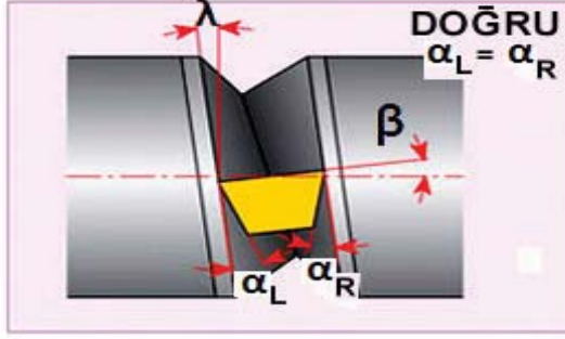
\alpha Yanal Temizleme Açısı
