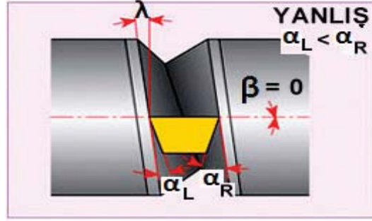
\lambda Helis (sarmal) Açısı
